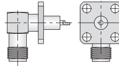
37. Right angle 4H jack
